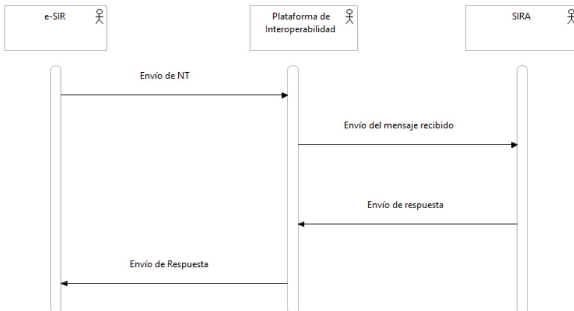
Figura 3: Diagrama de secuencia: Envío de NT por e-SIR
