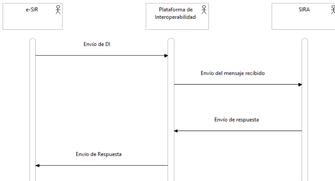
Figura 4: Diagrama de secuencia: Envío de DI por e-SIR
