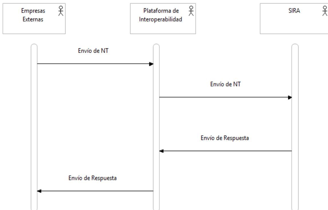
Figura 1: Diagrama de secuencia: Envío de NT por Empresa Externa
