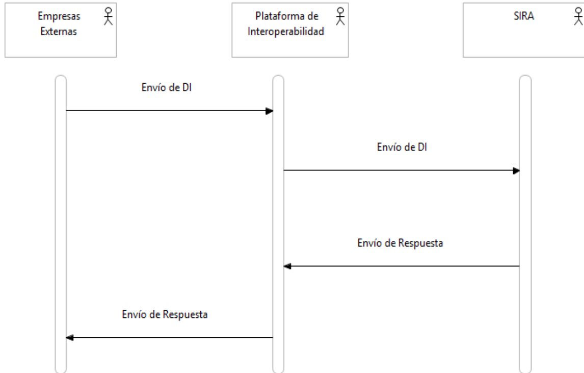
Figura 2: Diagrama de secuencia: Envío de DI por Empresa Externa
