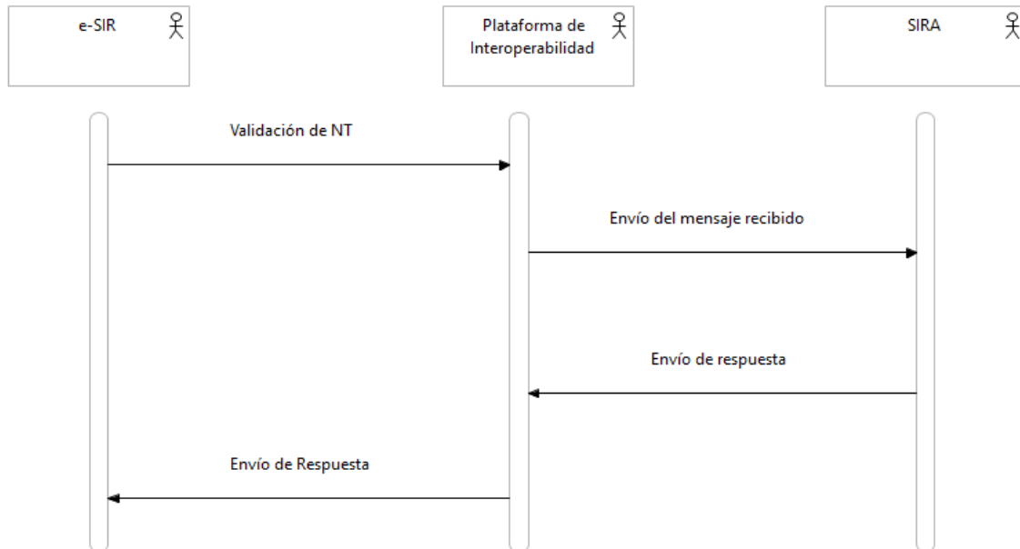
Figura 5: Diagrama de secuencia: Validación de NT por e-SIR
